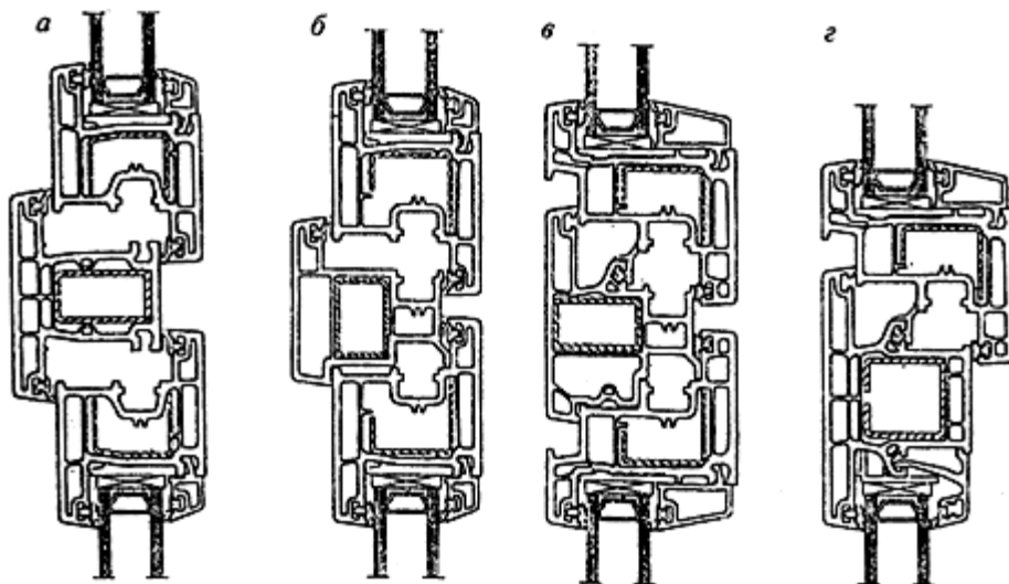
а - импостный притвор оконной системы с наружным и внутренним уплотнениями; б - штапловой (безимпостный) притвор оконной системы с наружным и внутренним уплотнениями; в - штапловой (безимпостный) притвор оконной системы со средним и внутренним уплотнениями; г - импостный притвор неоткрывающихся и открывающихся элементов оконной системы со средним и внутренним уплотнениями
